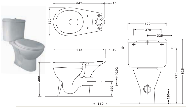
close coupled wc suite (lever flush)
