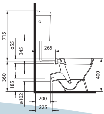
S7006011 - OL57 'P' Trap W.C. Pan
