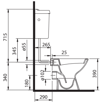
S7006010 - OL56 H.O. W.C. Pan
